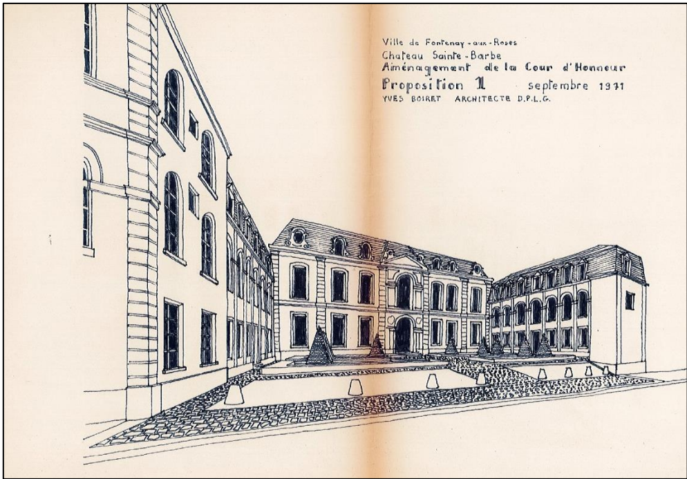
Ville de Fontenay-aux-Roses Chateau Sainte-Barbe Aménagement de la Cour d'Honneur Proposition II septembre 1931 YVES BOIRET ARCHITECTE D.P.L.G.
